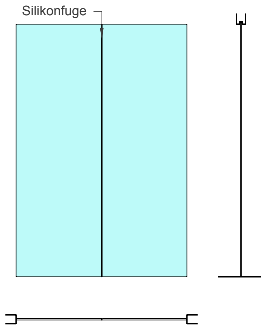
Ansicht und Schnitte
