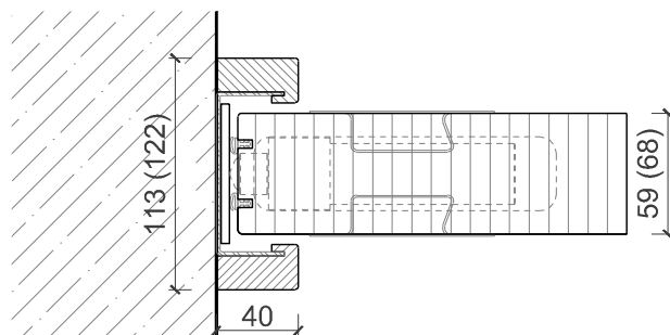
Anschlagprofil Wandaufliegend Einlauftiefe 33mm
