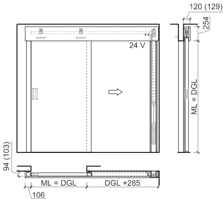
Anschlag (Horizontalschnitt)
