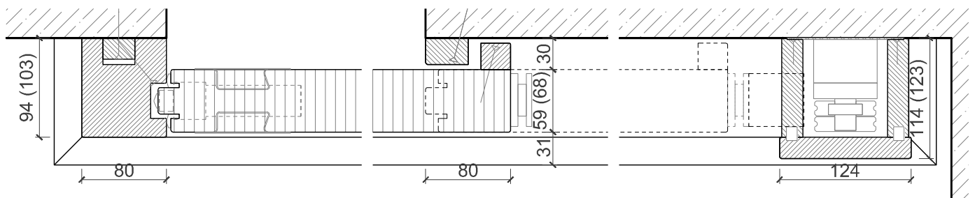
Anschlag (Horizontalschnitt)
