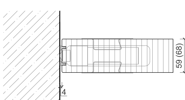
Ohne Anschlagprofil Stumpf gegen die Wand
